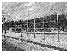
新金谷地区公民館に設置した 垂直型両面太陽光発電設備
