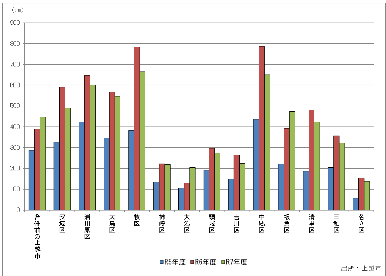
市内における累計降雪量の観測値 観測地点：合併前の上越市は高田特別地域気象観測所、13区は各区総合事務所
